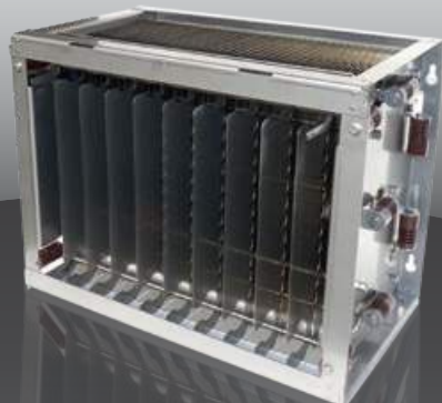
Abscheidetechnik: Elektrofilter
